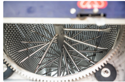
Un système d'égrappage horizontal
