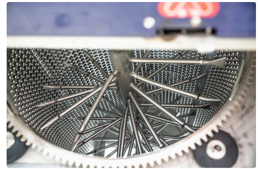
Un système d'égrappage horizontal
