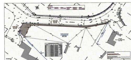
Plan des travaux effectué par Cédric Belestin, géomètre à Barcelonne-du-Gers et présenté au conseil municipal le 28 avril 2016.
