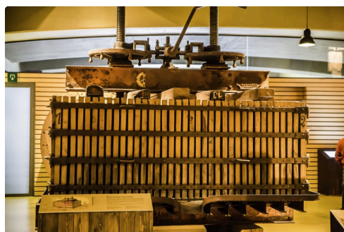
Pressoir à cage et à deux broches
